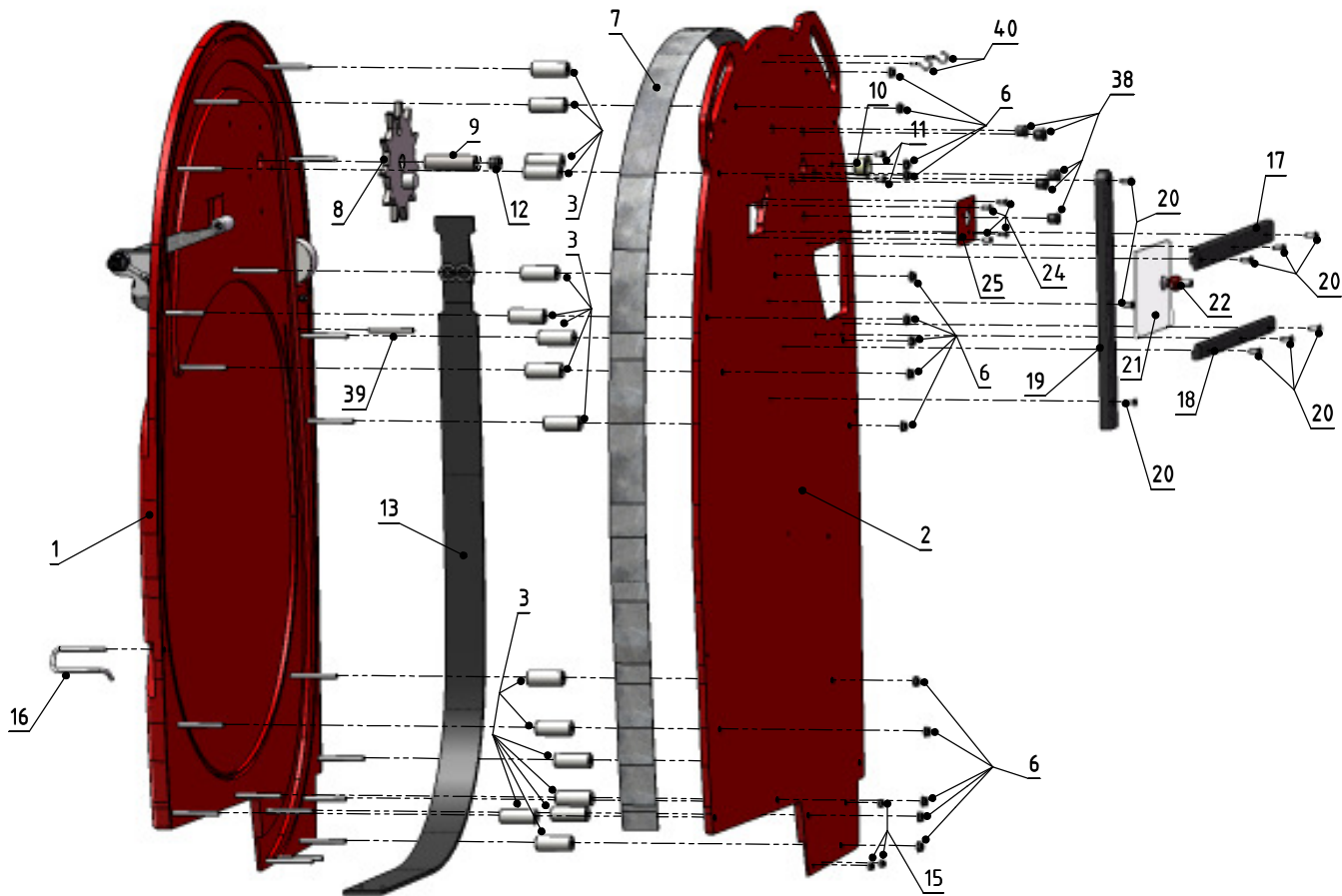
Speicherplatten Griffseite (Modell 700E/720E/730E) Storageplate handleside (Model 700E/720E730E)
