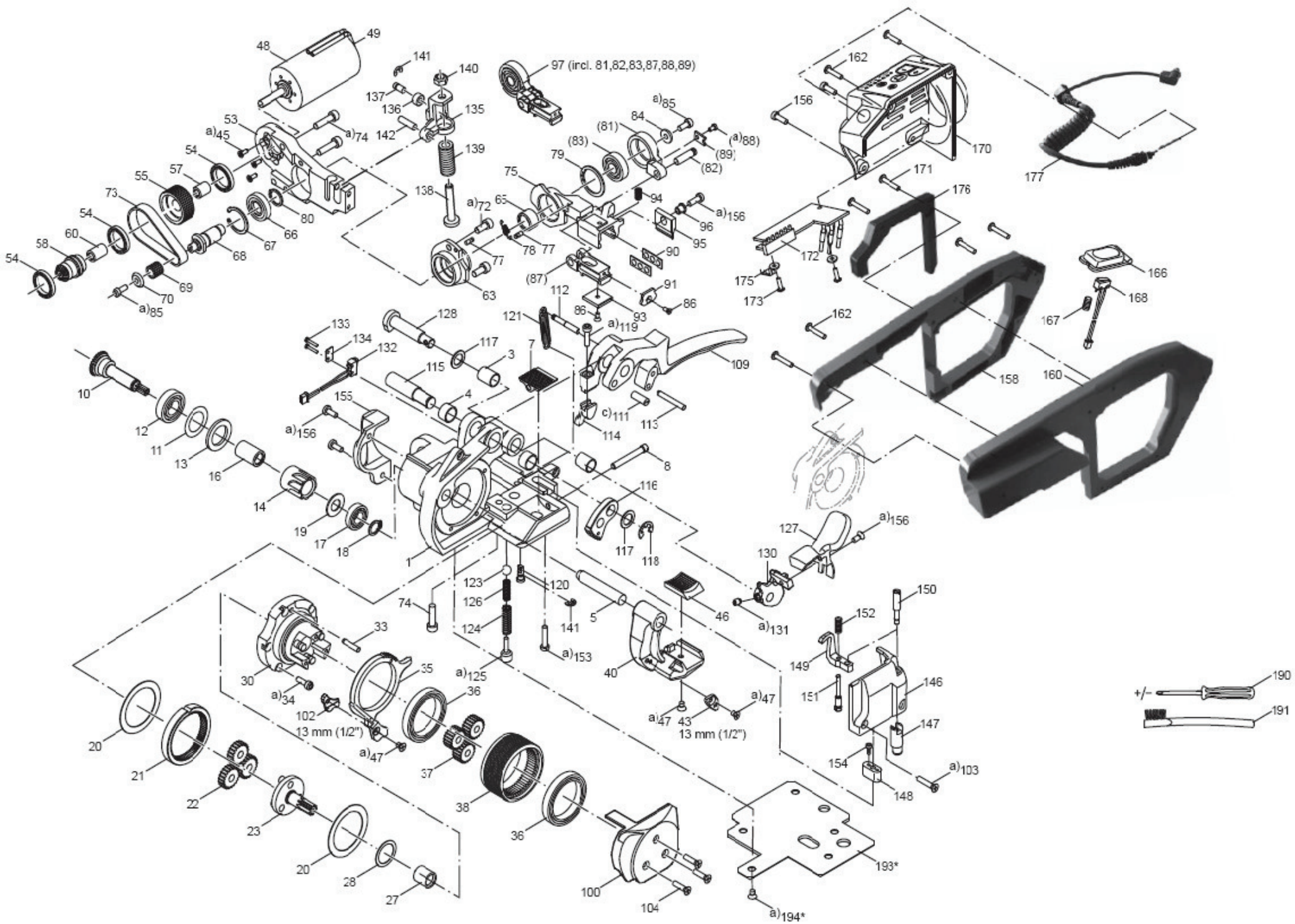
Verschlussgerät 720E / Locking tool 720E
